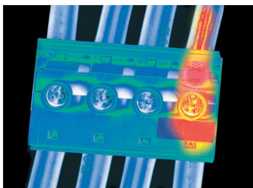
Sobrecarga del conductor neutro
