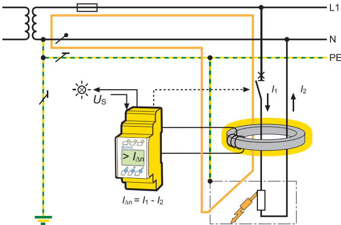
El principio de los sistemas RCM
